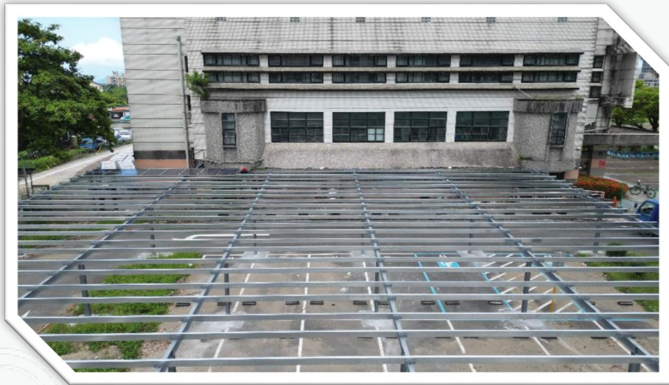
鋼構組立
